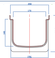
CANALETAS 200 REJILLAS METÁLICAS 200x500x188 2132201
