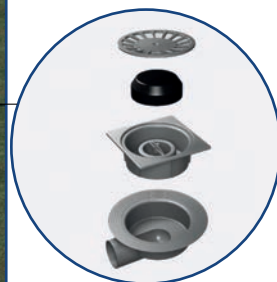
CALDERETA SIFÓNICA SALIDA HORIZONTAL
