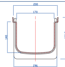
CANALETAS 200 PARA REJILLAS DE PP 200x500x188 1126630 y 1126638
