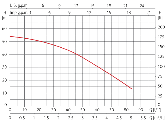
Curva de funcionamiento a 2900 rpm
