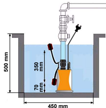
Dimensiones mínimas
